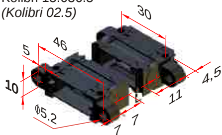
Kolibri 22.038.0 (Kolibri 05.0)
